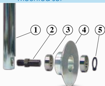
Cod. 313952 CONJUNTO MONTADO Mounted set
