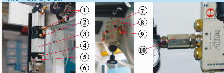
CILINDRO DOBLE CARRERA RP-30. Two Ways Cylinder
