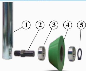
Cod. 313953 CONJUNTO MONTADO Mounted set
