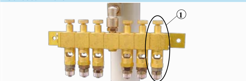
CONJUNTO VALVULAS PRIMER Outfeeds Primer Unit
