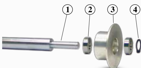
Cod. 294844 CONJUNTO MONTADO Mounted set
