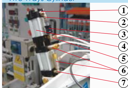
CILINDRO DOBLE CARRERA PL-32. Two Ways Cylinder
