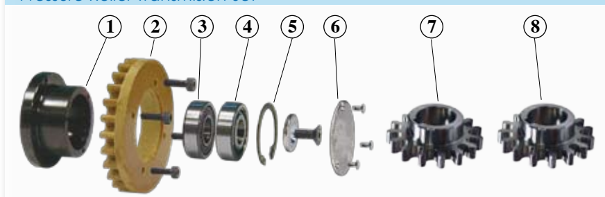
CONJUNTO TRANSMISIÓN ROD. PISÓN Pressure Roller Transmission Set
